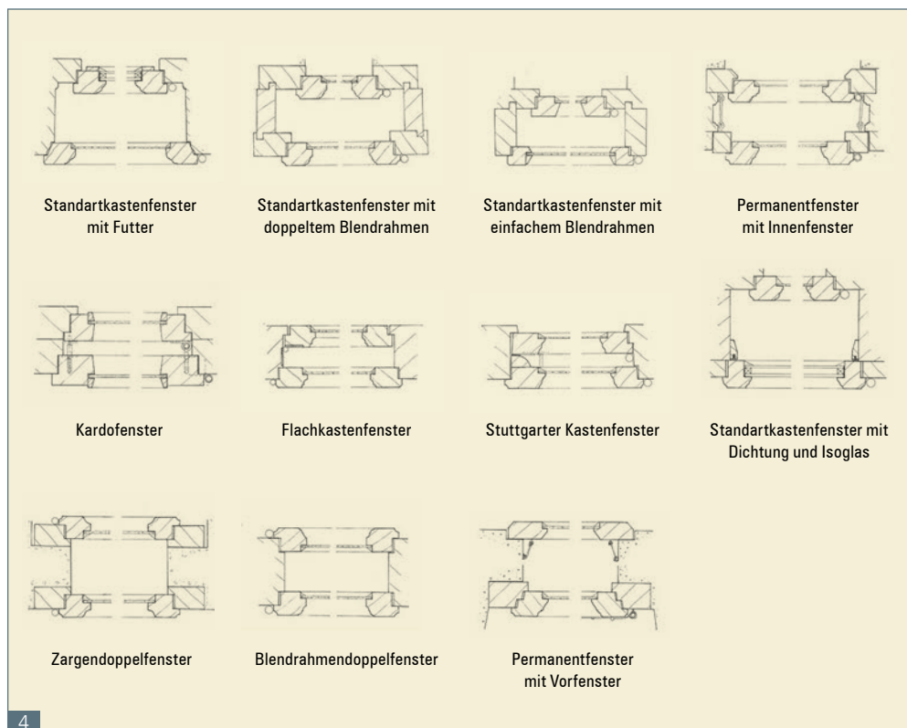
Abb. 4 Fenstergrundkonstruktionen. Die Darstellung zeigt die Vielfalt der möglichen zweischaligen Fenstervarianten.
