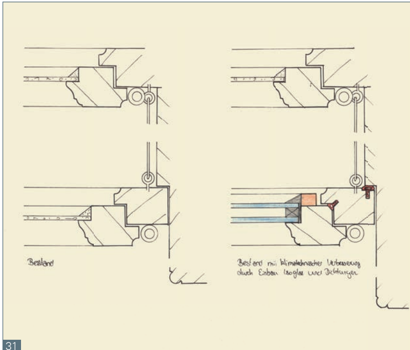
Abb. 31 Reutlingen, Seestraße 31. Zeichnerische Dokumentation des Fensterbestandes mit Detaillierung der energetischen Verbesserung.
