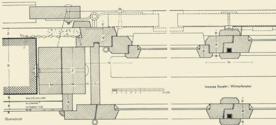
Drehflügel nach innen mit Lüftungsflügel nach innen, Blendrahmen, außen bündig
