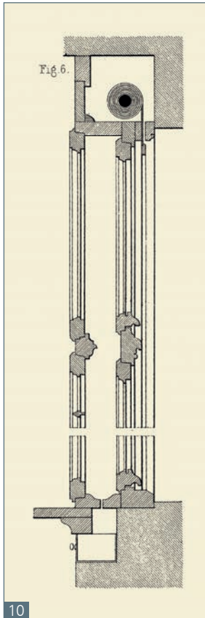
Abb. 10 Frühe Darstellung eines Kastenfensters mit Rollläden und Detaillierung einer Ent- wässerung im Sims zur Aufnah- me des Kondensats in einem unter dem Sims angebrachten Auffangbehälter.
